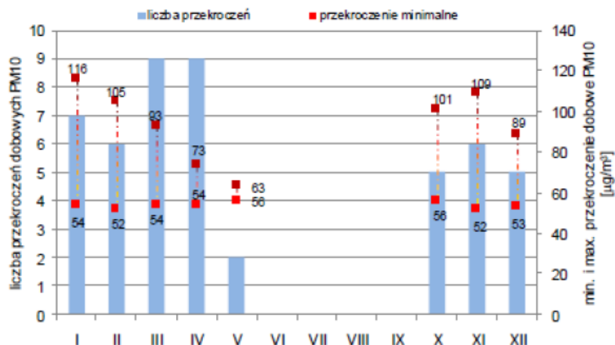
Rysunek 2. Liczba przekroczeń dobowych PM10 w Krośnie w 2013r. (źródło: Roczna Ocena Jakości Powietrza w województwie podkarpackim w 2013, WIOŚ Rzeszów).
